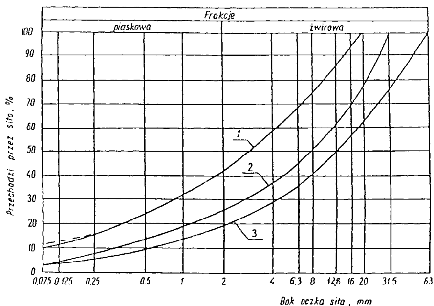
Rysunek 1. Pole dobrego uziarnienia kruszyw przeznaczonych na podbudowy wykonywane metodą stabilizacji mechanicznej 1-2 kruszywo na podbudowę zasadniczą (górną warstwę) lub podbudowę
